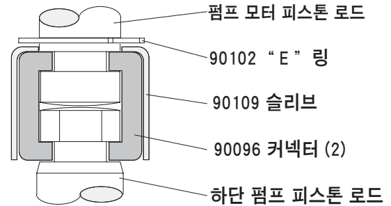
펌프 연결 세부도
